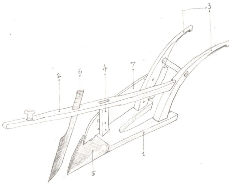
Fig. 3. Plug de construcție asimetrică. -- credit imagine Adrian Horațiu Pescaru 1. talpa plugului 2. grindeiul 3. coarnele 4. bârsa 5. brăzdarul 6. fierul lung 7. cormanul.
